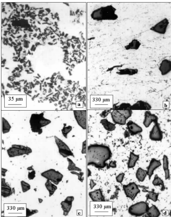
Figure 1: Composites RAR27 + Al_2O_3 , (OM); a) 3 mass %, 12\mu m , b) 3 mass %, 250\mu m , c) 8 mass %, 250\mu m , d) 16 mass %, 250\mu m
